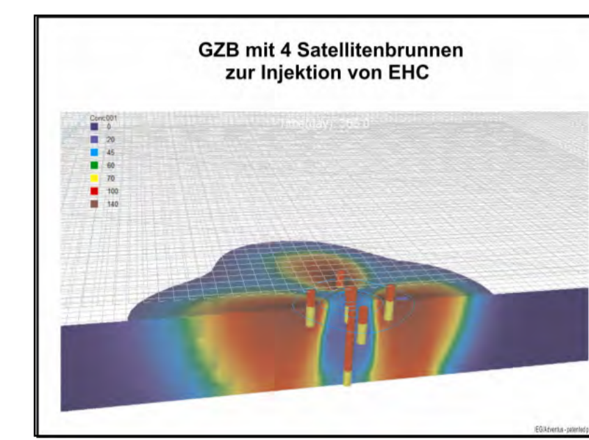
GZB mit 4 Satellitenbrunnen zur Injektion von EHC
