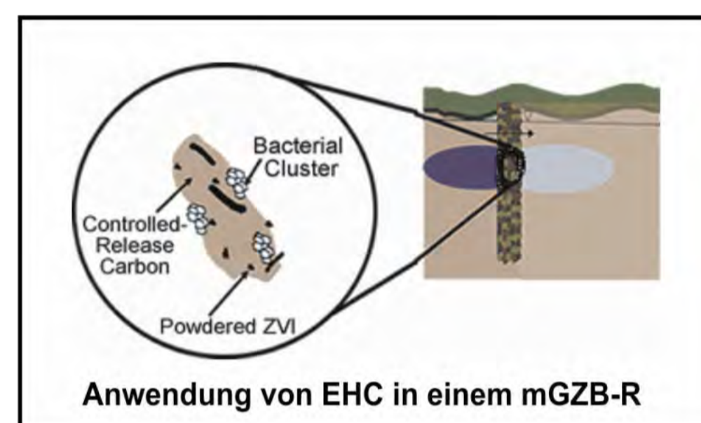
Anwendung von EHC in einem mGZB-R
