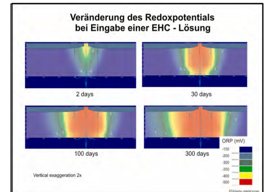
Veränderung des Redoxpotentials bei EHC - Lösung
