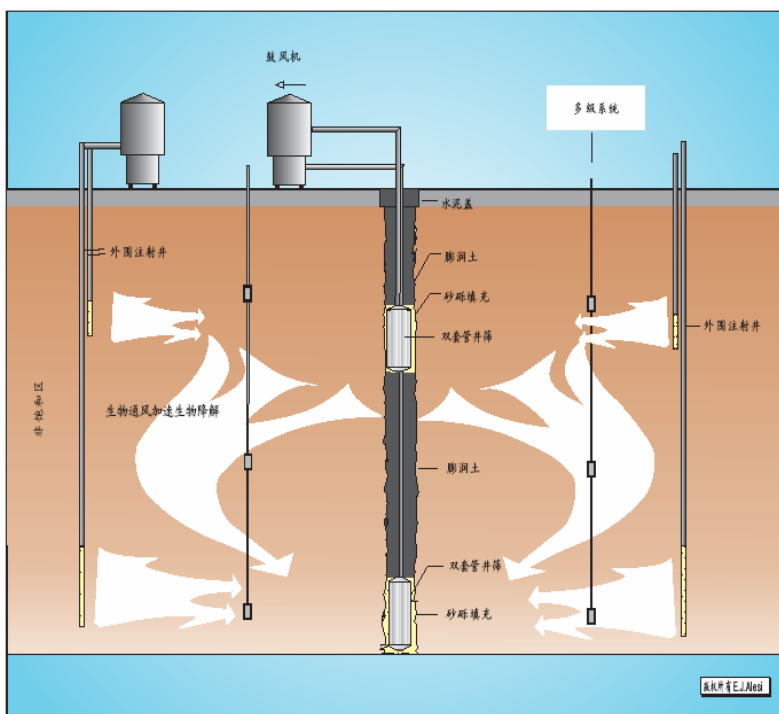
土壤气体循环-生物通风-生物降解去除非挥发性污染物 (IEG SAC-生物通风技术)
